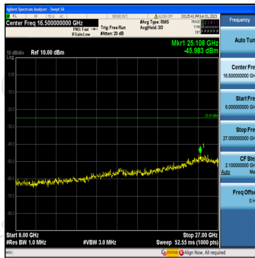
Band7-10MHz-QPSK-20800-50RB#0-Range3:6000~27000MHz
