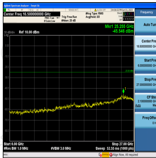
Band7-20MHz-QPSK-21350-100RB#0-Range3:6000~27000MHz
