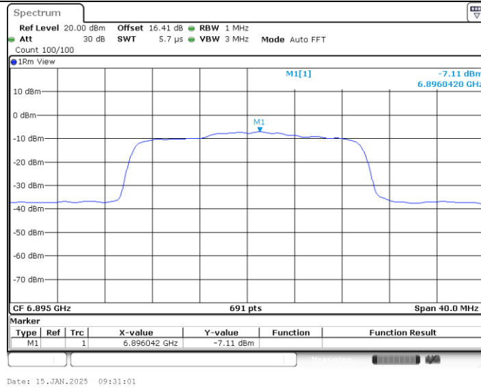
11AX20MIMO_Ant2_6895
