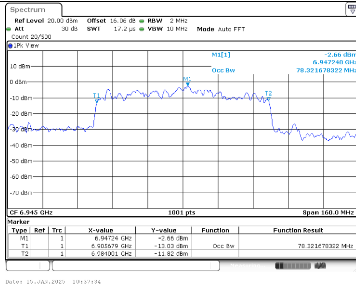
11AX80MIMO_Ant2_6945
