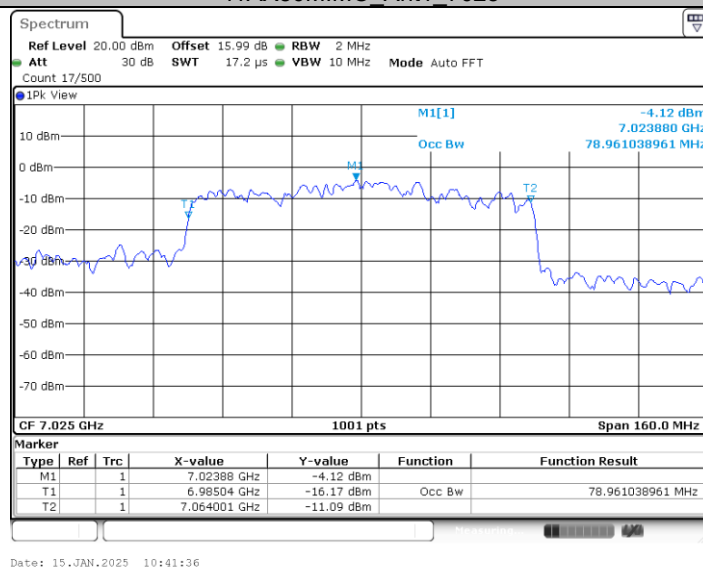
11AX80MIMO_Ant2_7025
