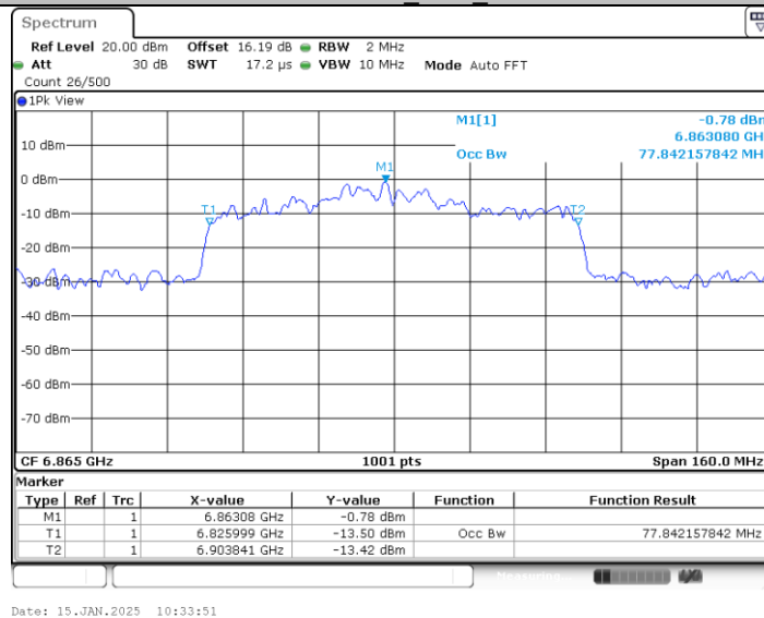
11AX80MIMO_Ant2_6865
