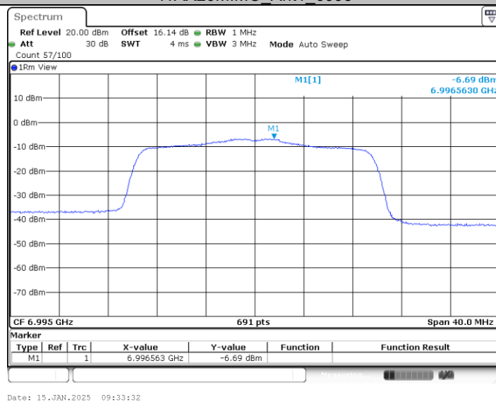
11AX20MIMO_Ant2_6995
