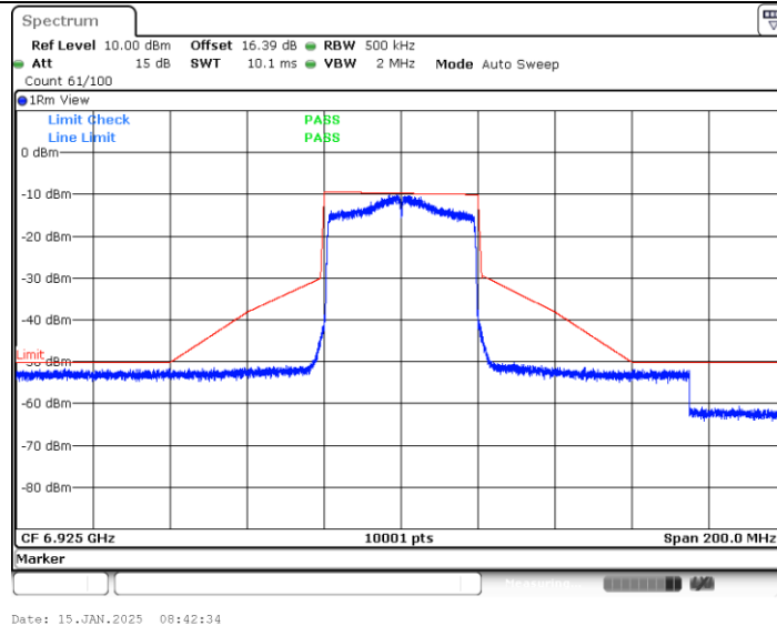
11AX40MIMO_Ant2_6925
