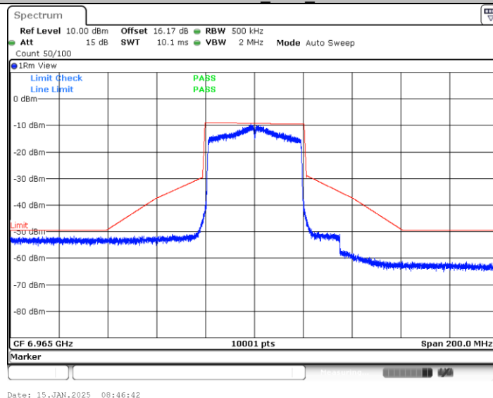
11AX40MIMO_Ant2_6965
