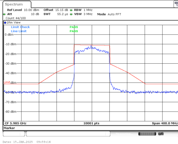
11AX80MIMO_Ant2_5985
