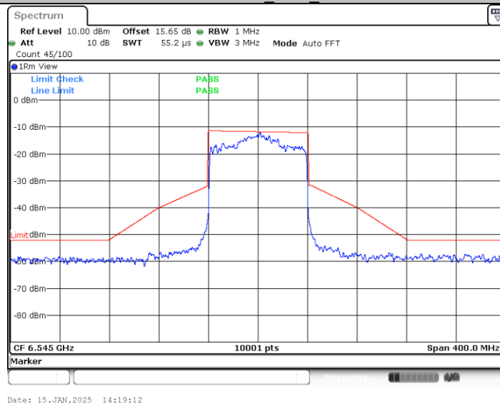
11AX80MIMO_Ant2_6545
