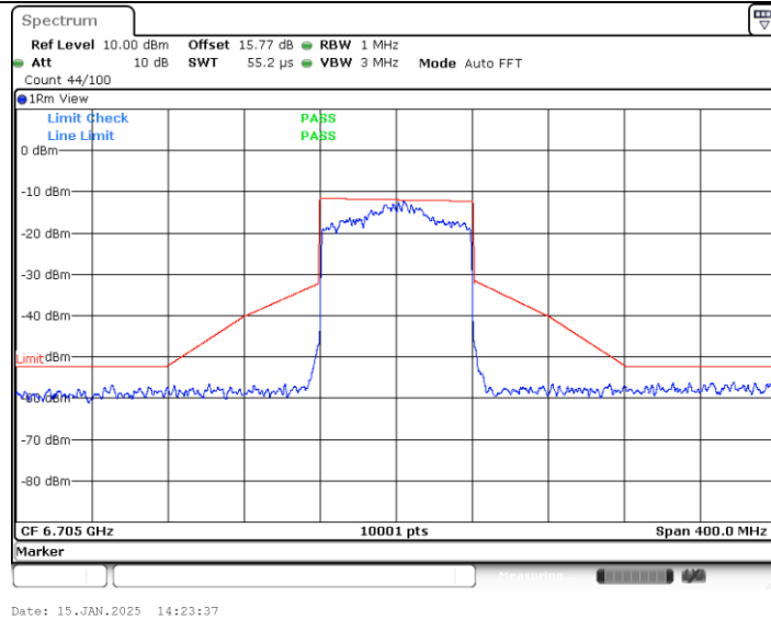
11AX80MIMO_Ant2_6705
