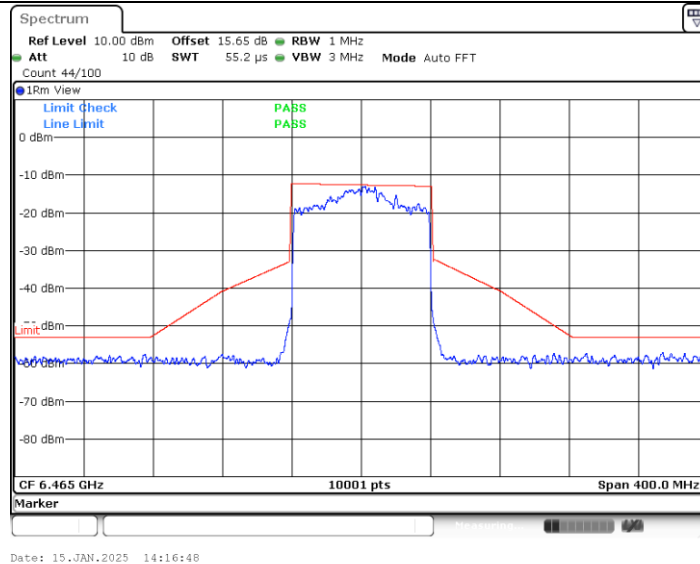
11AX80MIMO_Ant2_6465
