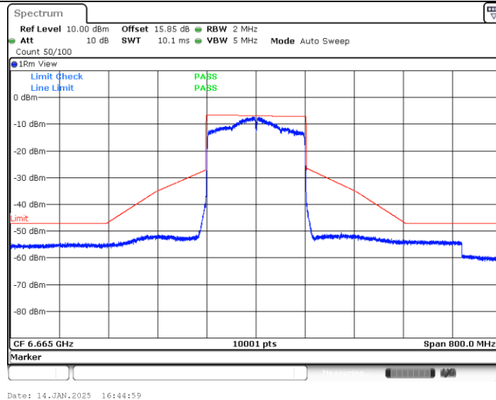
11AX160MIMO_Ant2_6665
