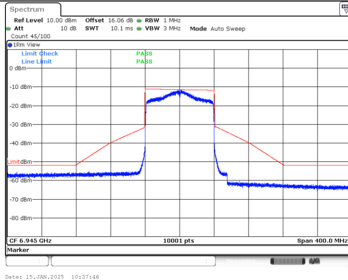
11AX80MIMO_Ant2_6945
