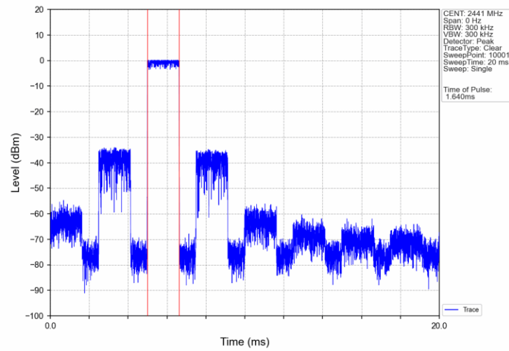
GFSK_DH3_HOPP_Ant1_NTNV
