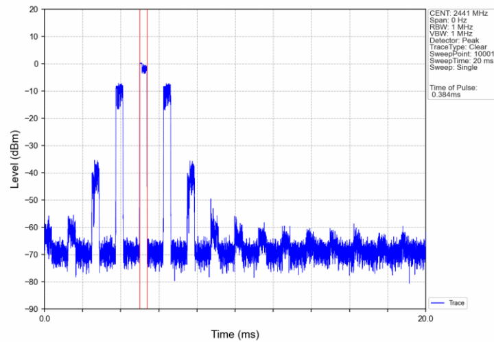
8DPSK_3DH1_HOPP_Ant1_NTNV
