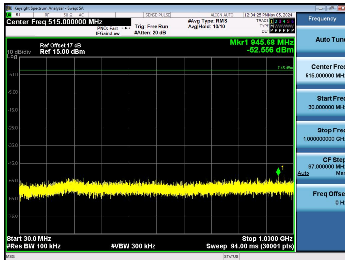
2.4G-Ant2-2479.4-30~1000-PASS
