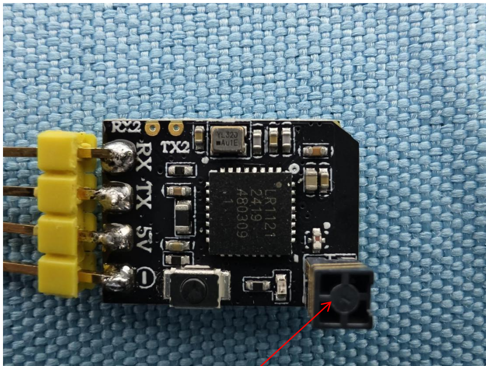
2.4G-ANT
