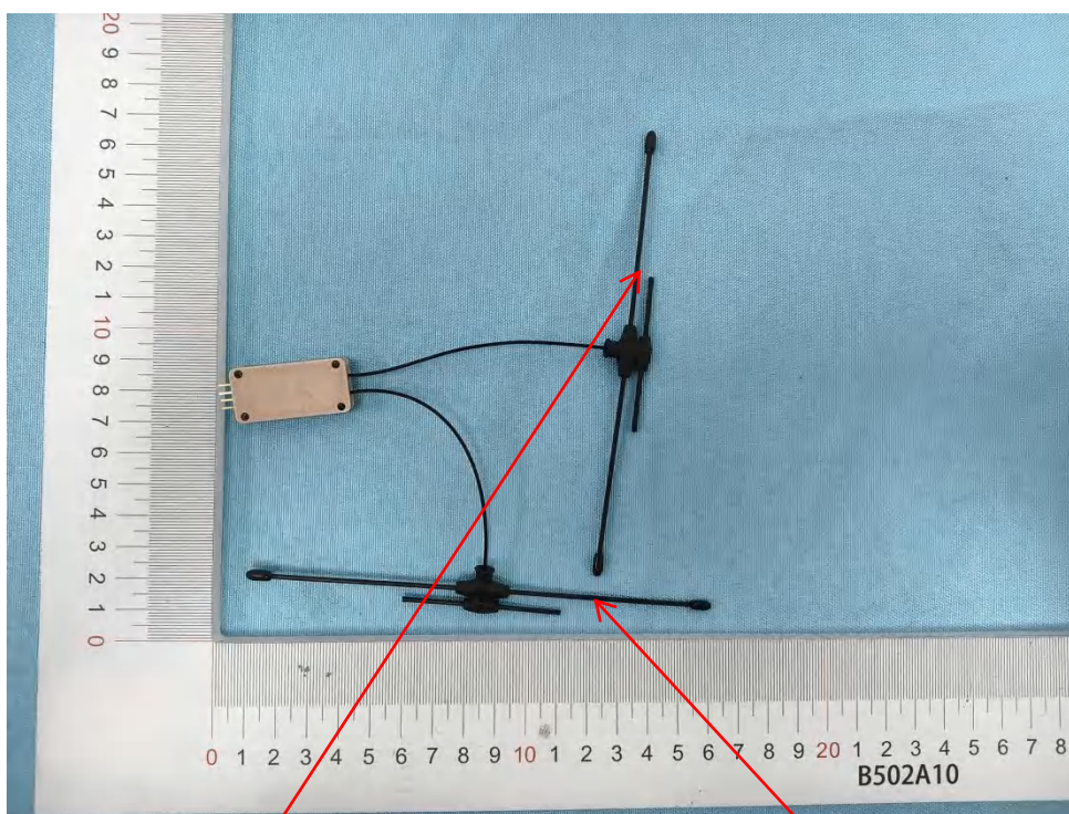
2.4G&900MHz-ANT1
