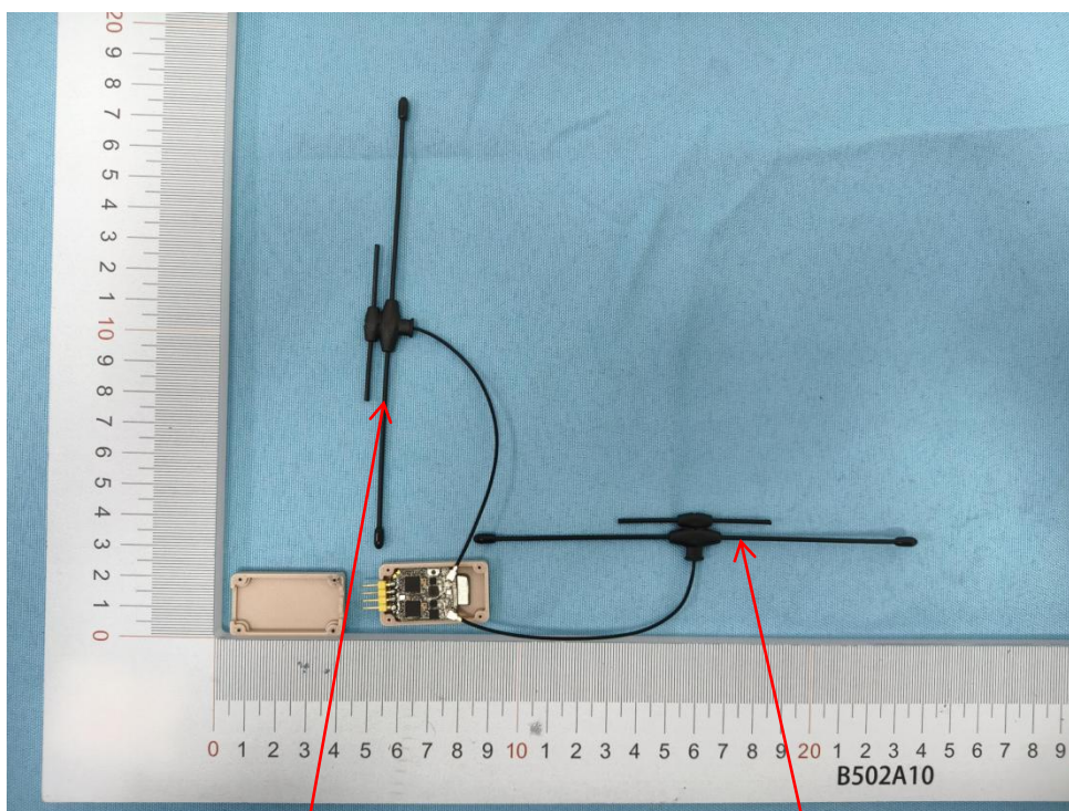
2.4G&900MHz-ANT1
