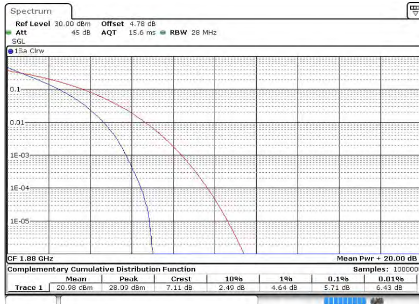
Band2-20MHz-QPSK-18900-100RB#0
