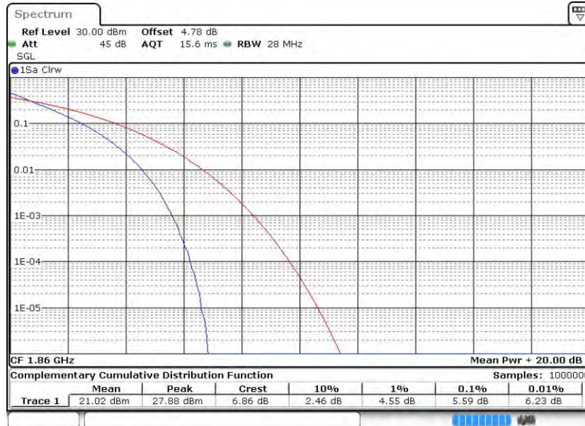
Band2-20MHz-QPSK-18700-100RB#0
