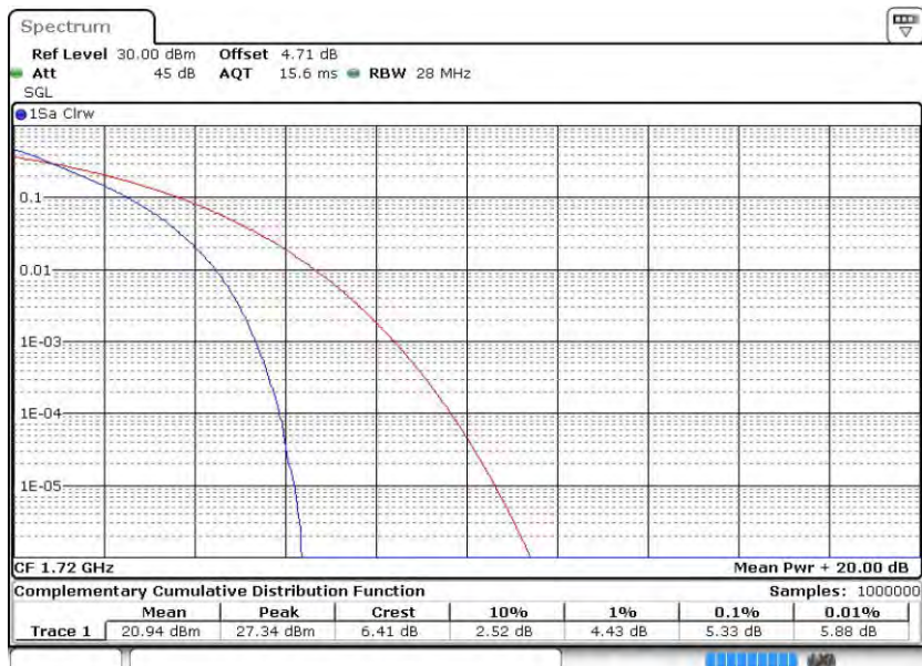
Band4-20MHz-QPSK-20050-100RB#0
