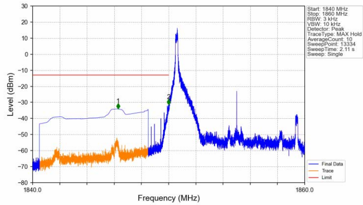
Band2_10MHz_QPSK_LCH_1855MHz_RB_1_0_NTNV
