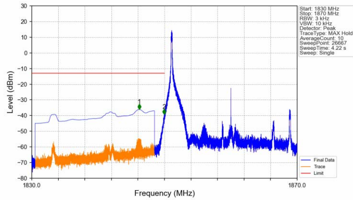
Band2_20MHz_QPSK_LCH_1860MHz_RB_1_0_NTNV
