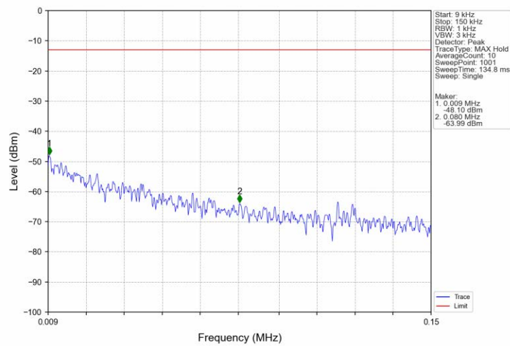
Band66_20MHz_QPSK_LCH_1720MHz_RB_1_0_NTNV
