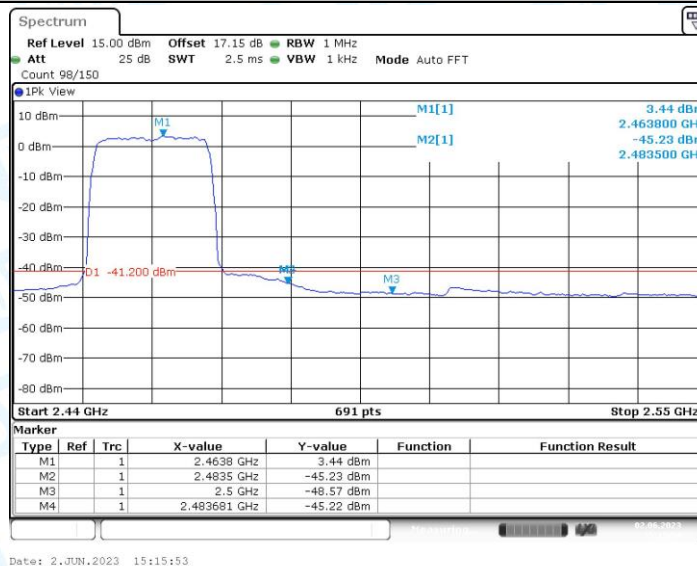
11N20MIMO_Ant1_High_2462_AV
