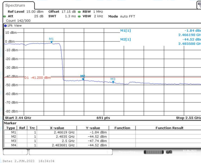
11AX40MIMO_Ant1_High_2452_AV
