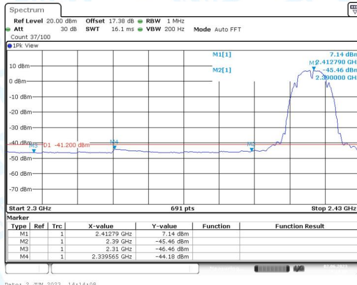
11B-CDD_Ant1_Low_2412_AV
