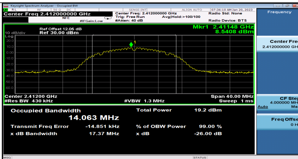
11B Ant1 2412
