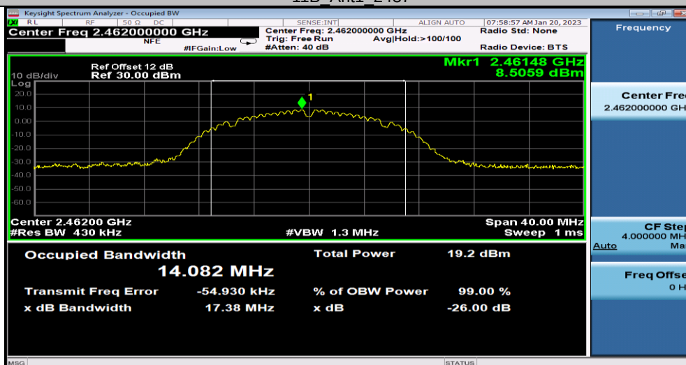
11B Ant1 2462
