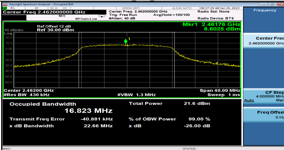
11G_Ant1_2462
