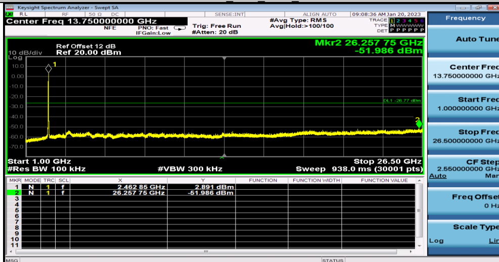
11N20SISO Ant1 2462 1000~26500
