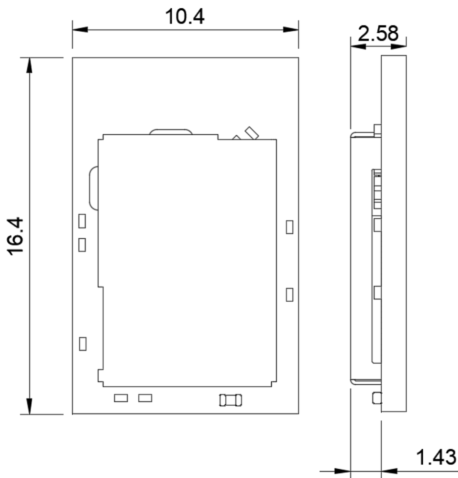
Fig 2.1.1 PCB dimensions
