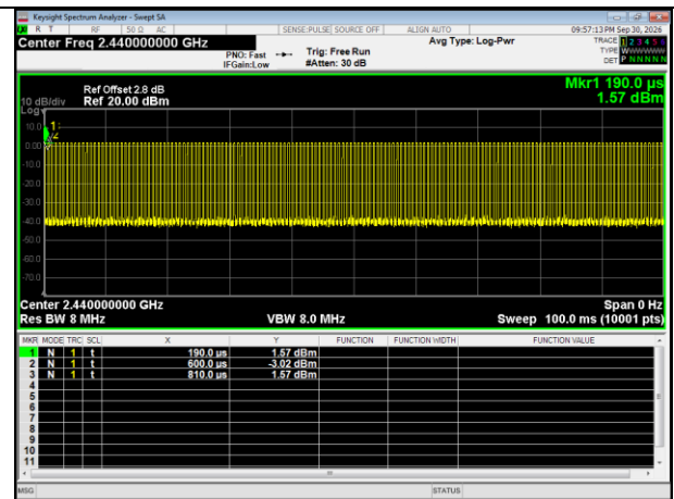
BLE 2M_Channel 19
