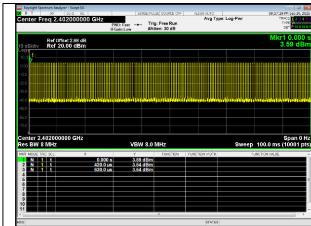
BLE 2M_Channel 0
