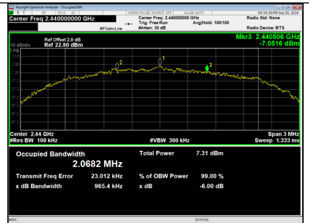
BLE 2M_Channel 19
