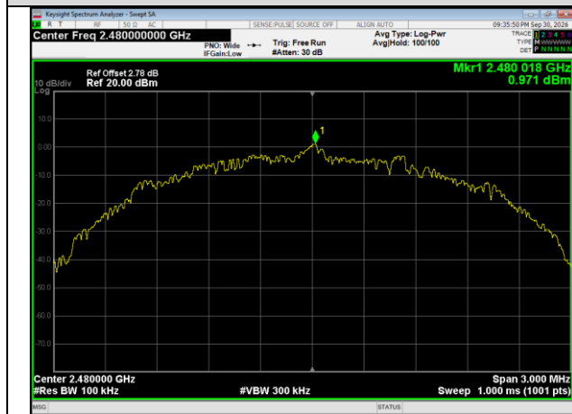
BLE 2M_Channel 39
