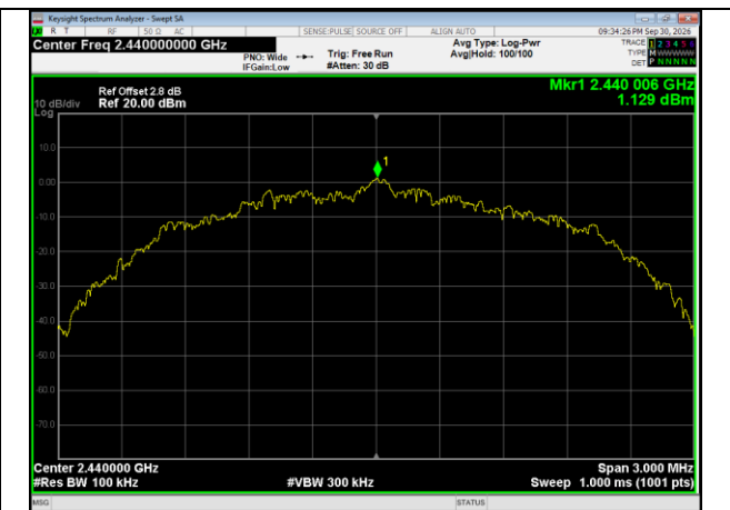
BLE 2M_Channel 19
