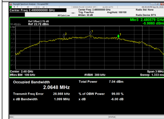
BLE 2M_Channel 39
