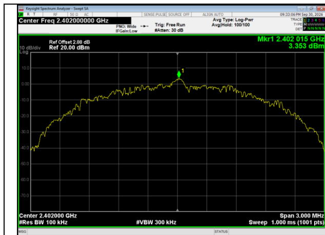
BLE 2M_Channel 0
