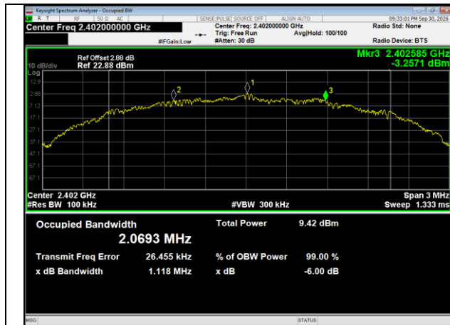
BLE 2M_Channel 0
