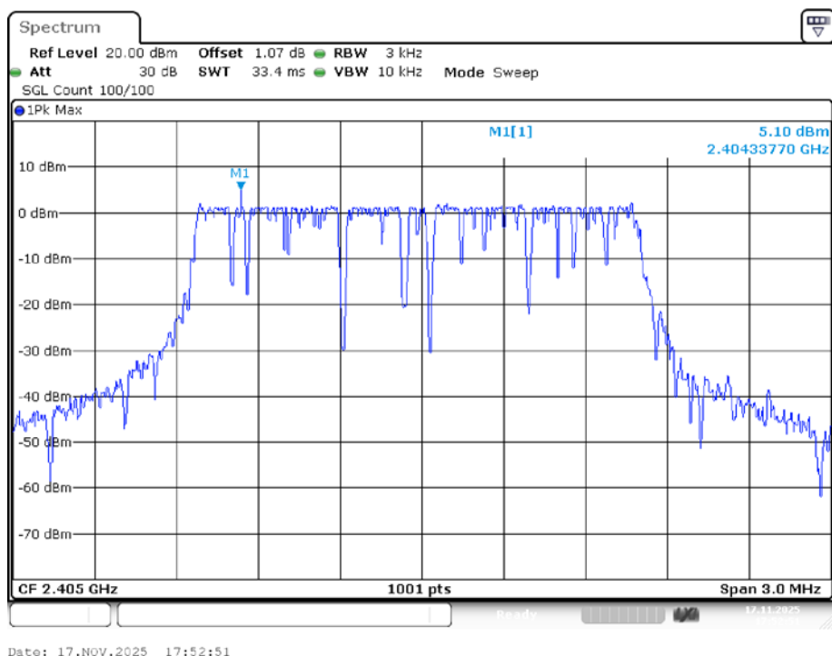
PSD NVNT LORA 2405MHz Ant1
