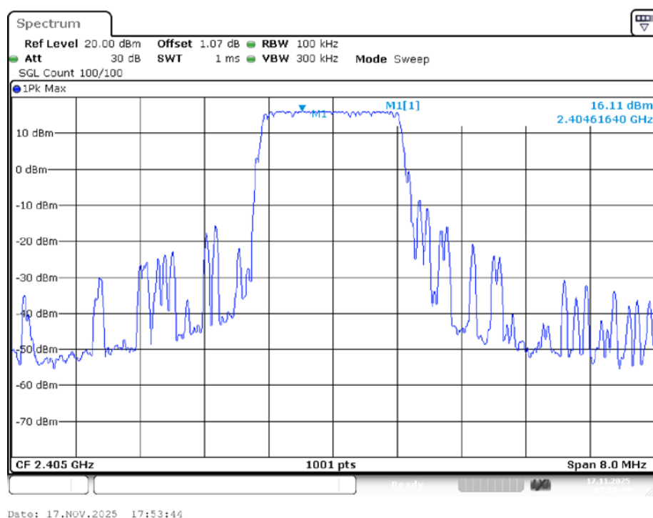
Band Edge NVNT LORA 2405MHz Ant1 Ref
