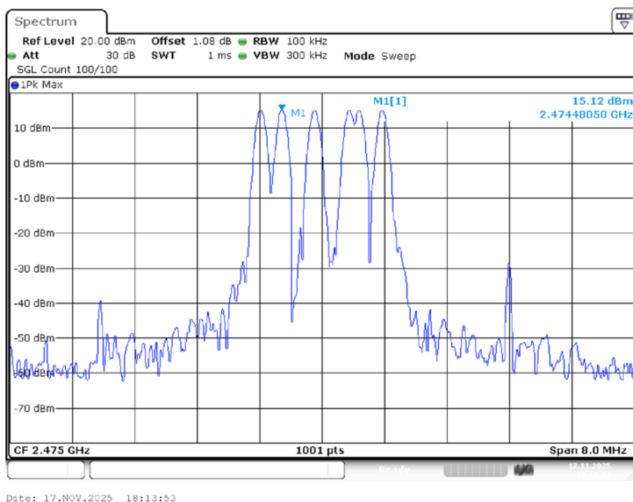
Band Edge NVNT LORA 2475MHz Ant1 Ref
