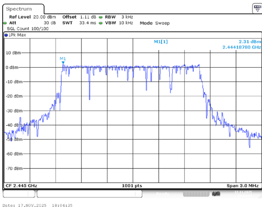
PSD NVNT LORA 2445MHz Ant1
