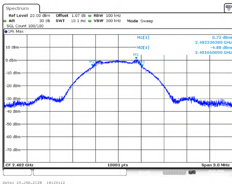
-6dB Bandwidth NVNT BLE 1M 2402MHz Ant1
