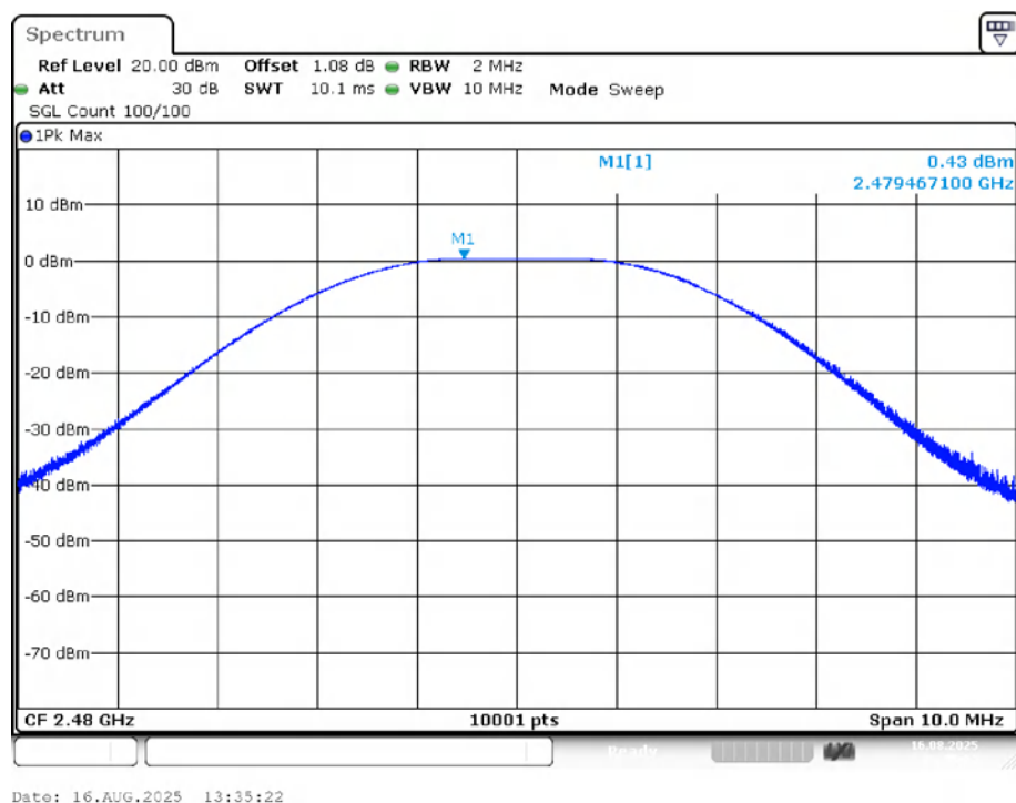
Power NVNT BLE 2M 2480MHz Ant1
