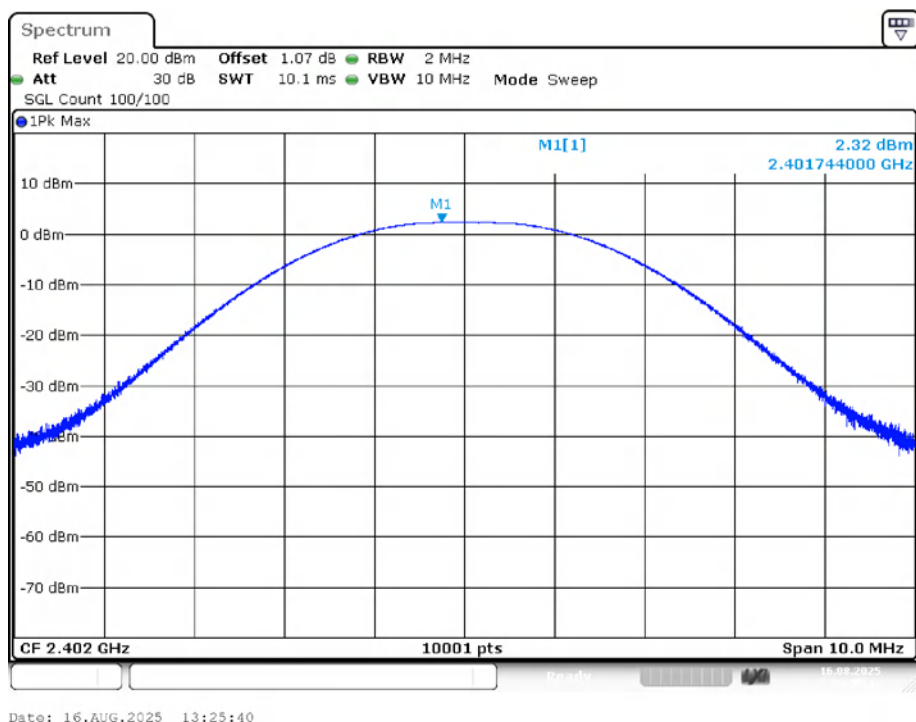
Power NVNT BLE 1M 2402MHz Ant1
