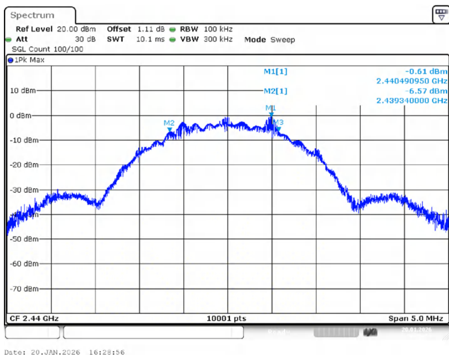
-6dB Bandwidth NVNT BLE 2M 2440MHz Ant1
