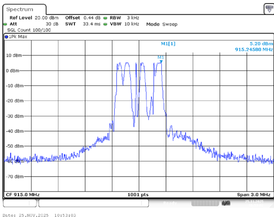
PSD NVNT LORA 915MHz Ant1
