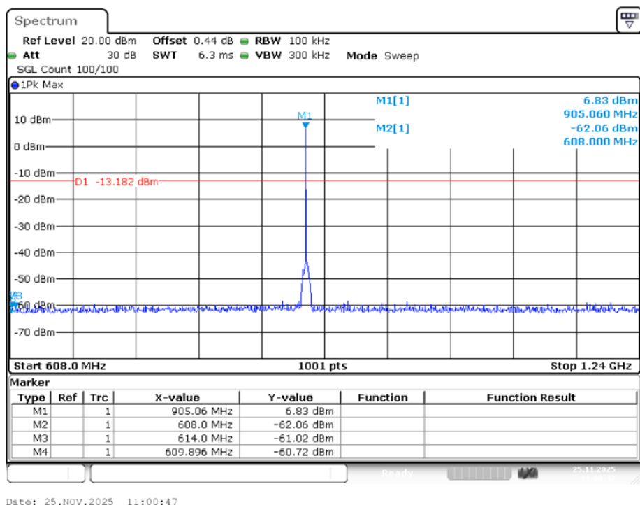
Band Edge NVNT LORA 905MHz Ant1 Emission
