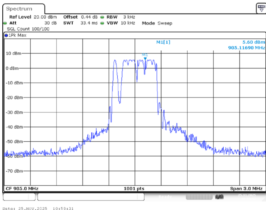
PSD NVNT LORA 905MHz Ant1
