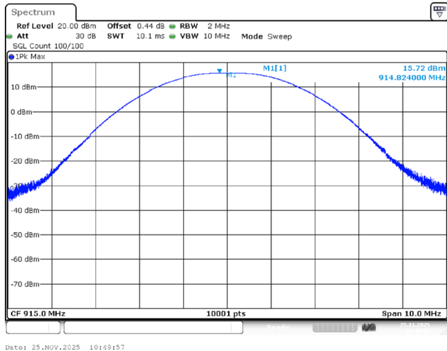
Power NVNT LORA 915MHz Ant1
