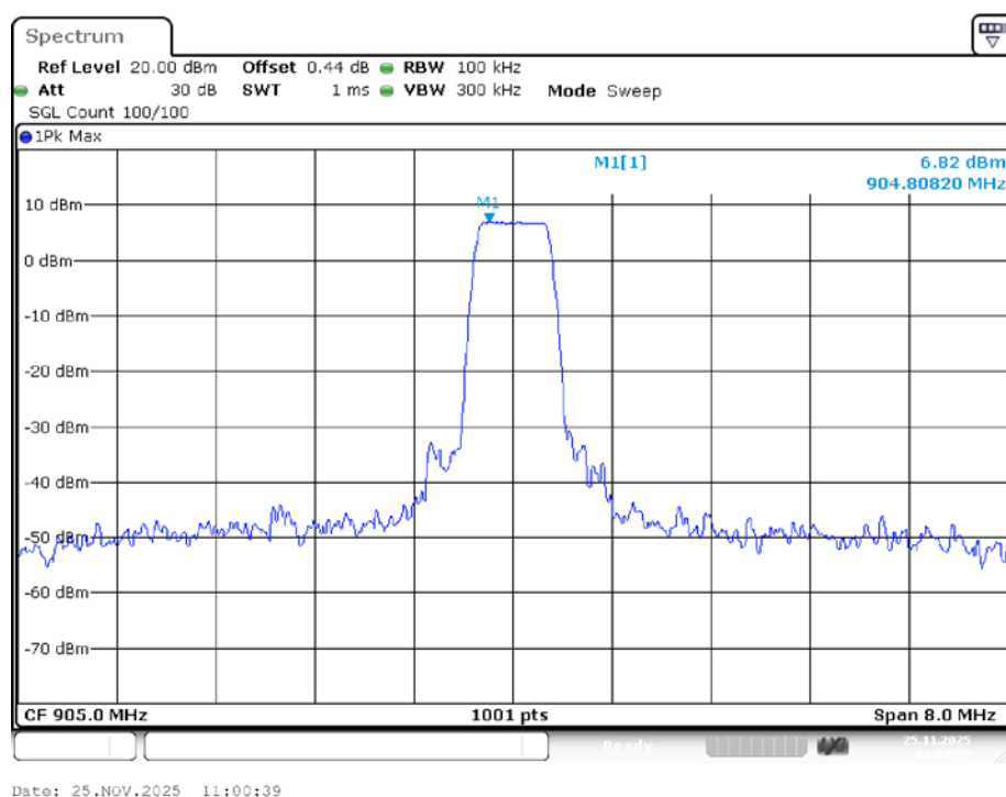
Band Edge NVNT LORA 905MHz Ant1 Ref
