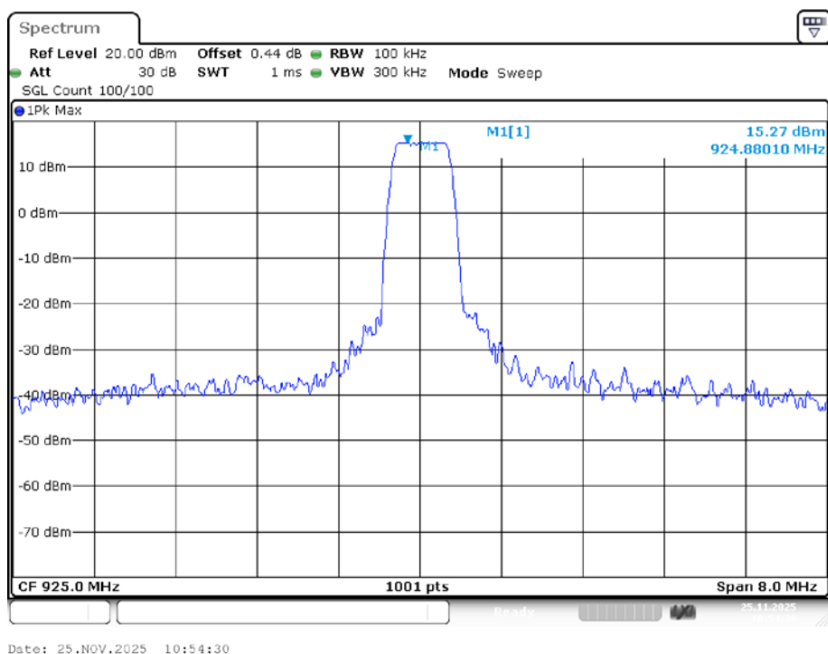
Band Edge NVNT LORA 925MHz Ant1 Ref
