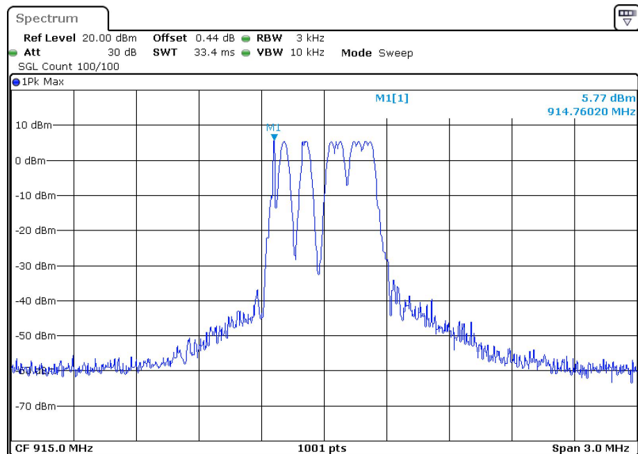
PSD NVNT LORA 915MHz Ant1
