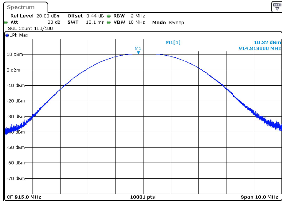
Power NVNT LORA 915MHz Ant1
