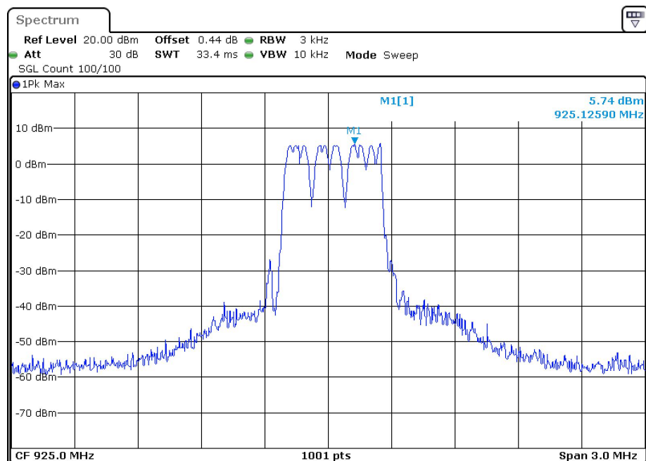
PSD NVNT LORA 925MHz Ant1
