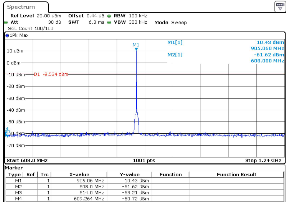
Band Edge NVNT LORA 905MHz Ant1 Emission
