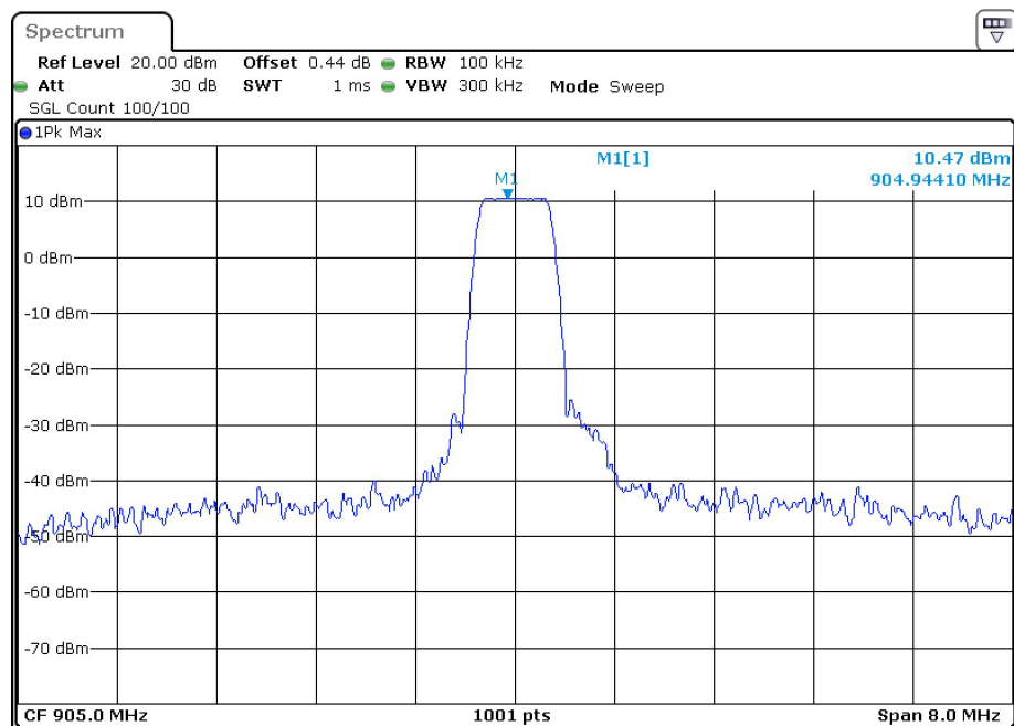
Band Edge NVNT LORA 905MHz Ant1 Ref
