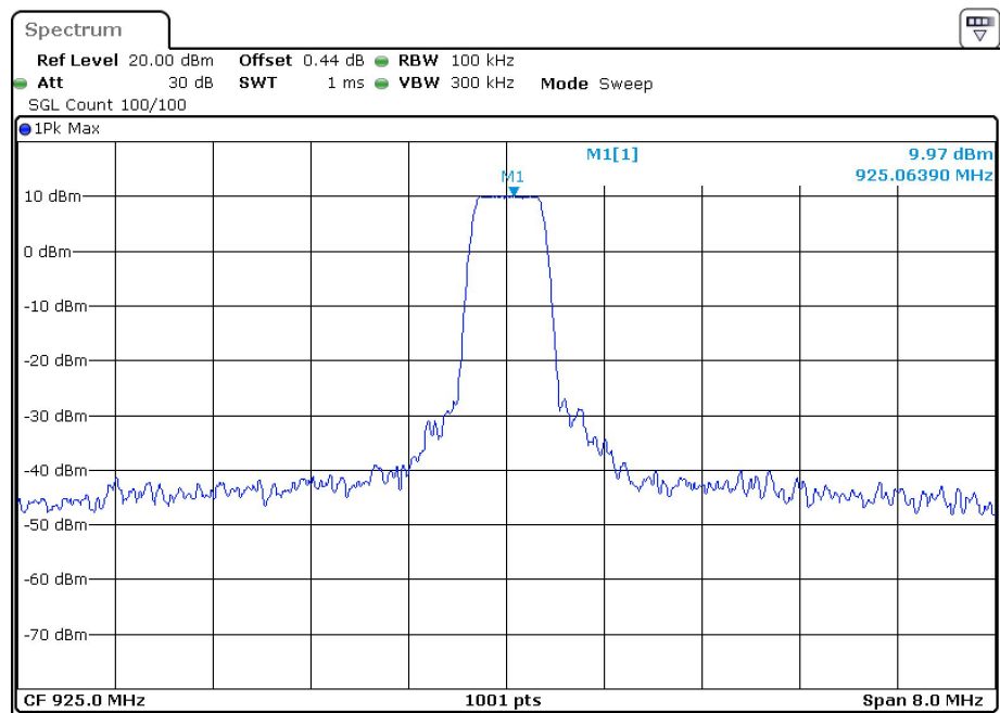
Band Edge NVNT LORA 925MHz Ant1 Ref
