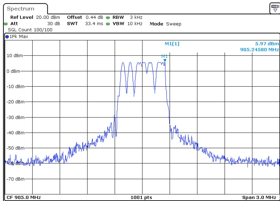
PSD NVNT LORA 905MHz Ant1
