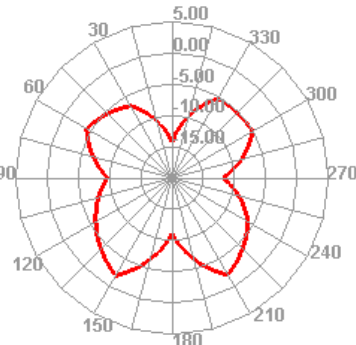
2400.000MHz E2
