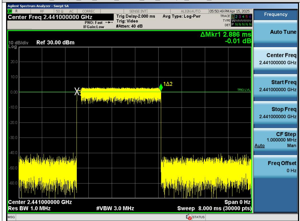
Test_Graph_BR_HOP_ANT1_NA_2Mbps_2441_Time per Burst
