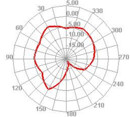
5150.000MHz E2
