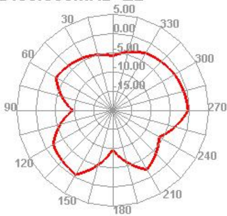
2450.000MHz E2
