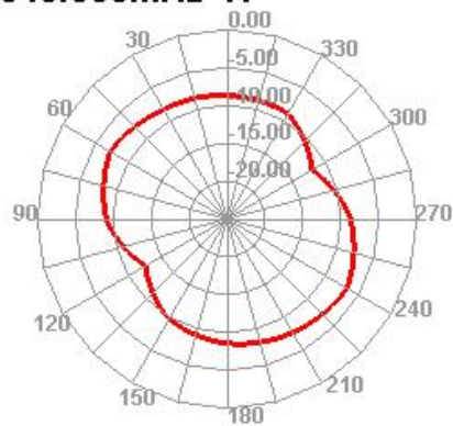
840.000MHz H
