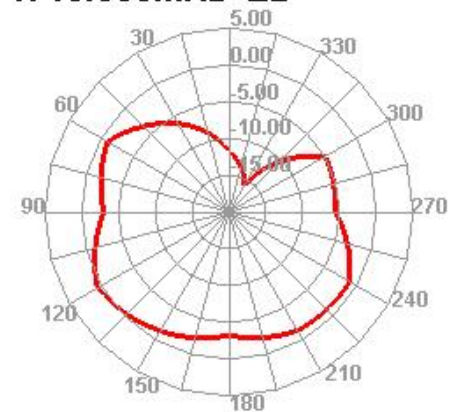
1710.000MHz E2
