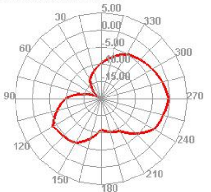
2450.000MHz H
