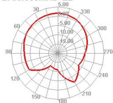
2700.000MHz E2
