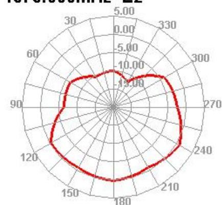
1575.000MHz E2
