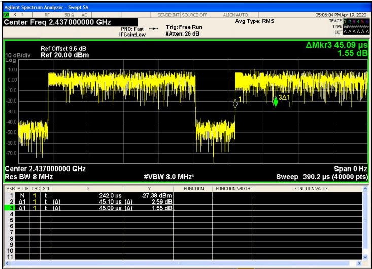
IEEE 802.11n_20MHz_Channel 6
