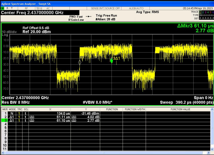
IEEE 802.11n_40MHz_Channel 6
