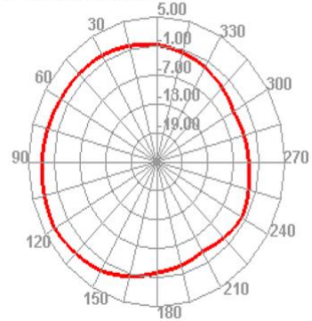
2450.000MHz H
