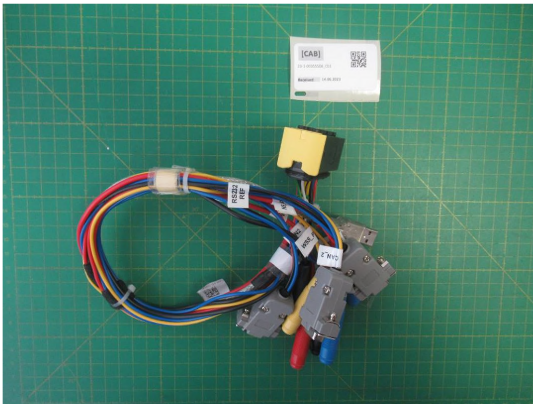
Fig. Ext.: 8 : Ext. - Front USB cable CAB 2
