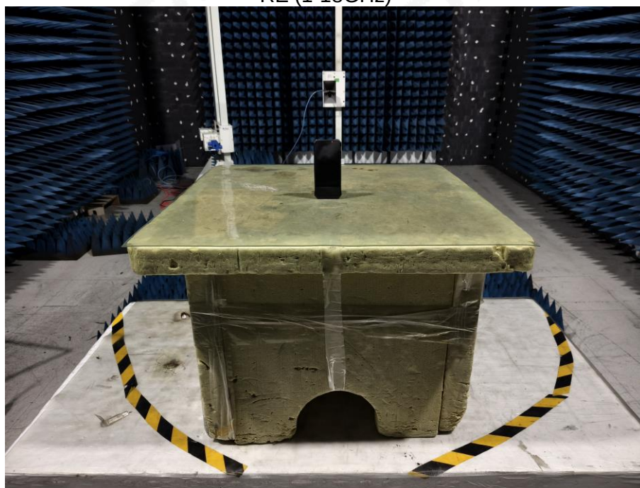
RE (1-18GHz)
