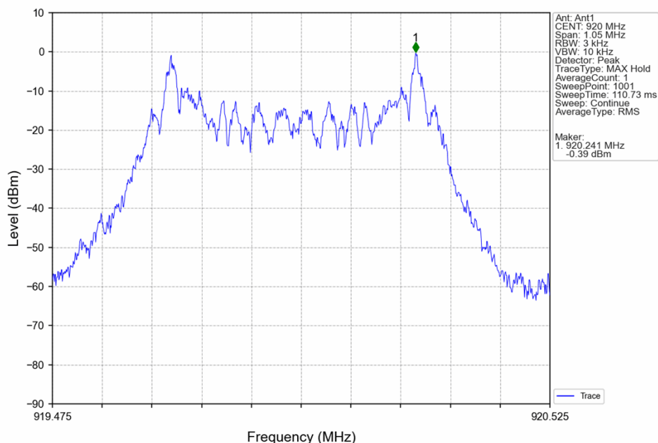
HCH_920MHz_Ant1_NTNV
