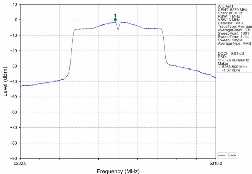
802.11n(HT40)_LCH_5270MHz_Ant1_NTNV
