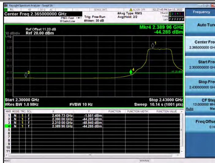
11N20SISO_Ant1_Low_2412_AV
