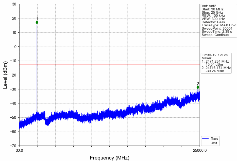
1.4M_HCH_2471.12MHz_Ant2_NTNV
