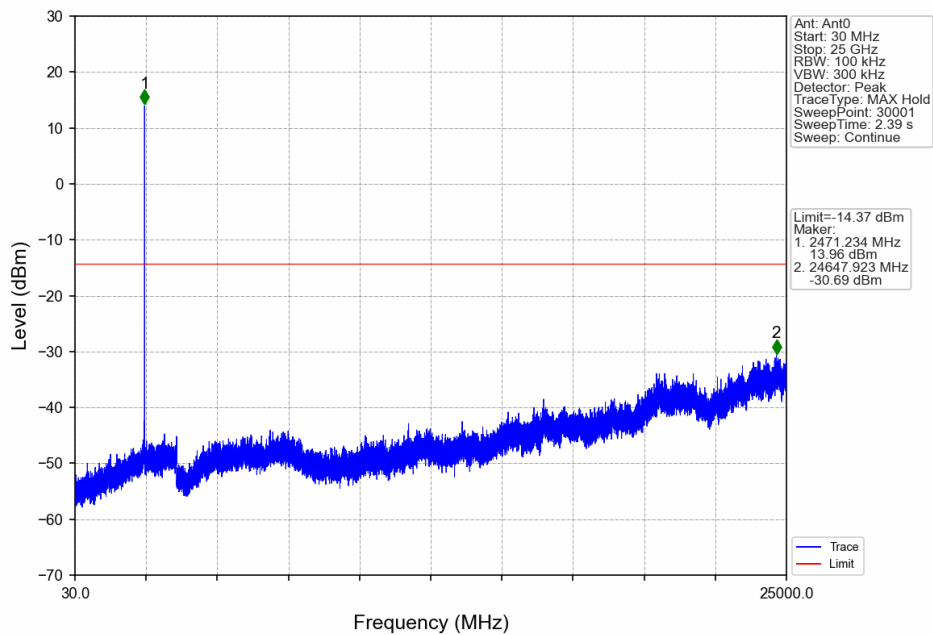
3M_HCH_2471.2MHz_Ant0_NTNV
