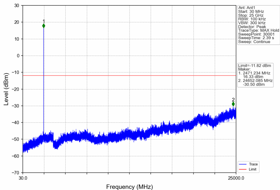
1.4M_HCH_2471.12MHz_Ant1_NTNV
