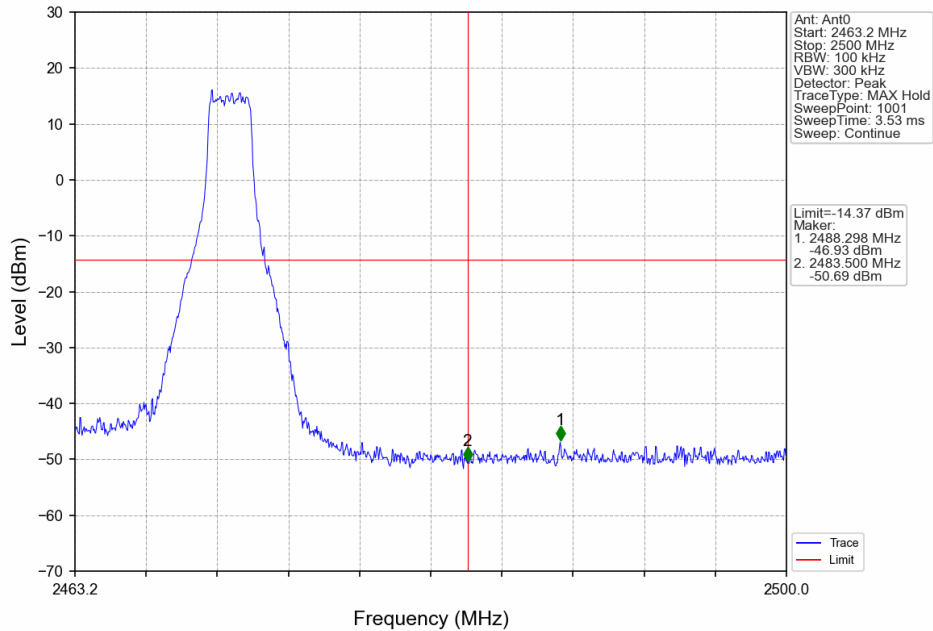
3M_HCH_2471.2MHz_Ant0_NTNV
