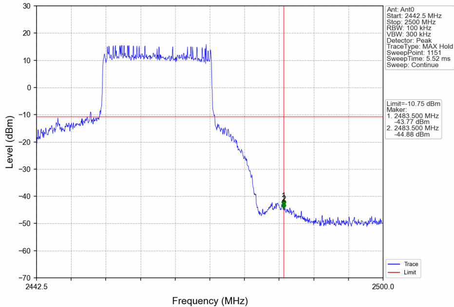
20M_HCH_2462.5MHz_Ant0_NTNV
