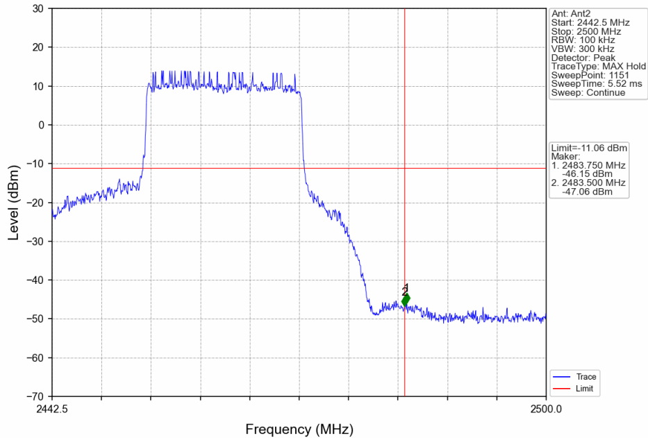
20M_HCH_2462.5MHz_Ant2_NTNV
