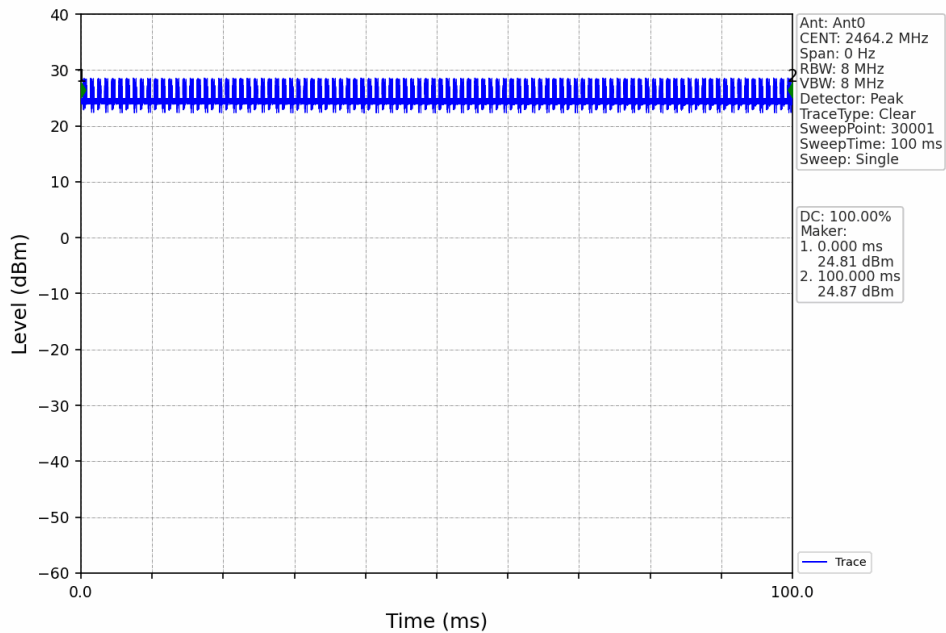
3M_HCH_2464.2MHz_Ant0_NTNV
