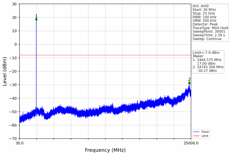
3M_HCH_2464.2MHz_Ant0_NTNV
