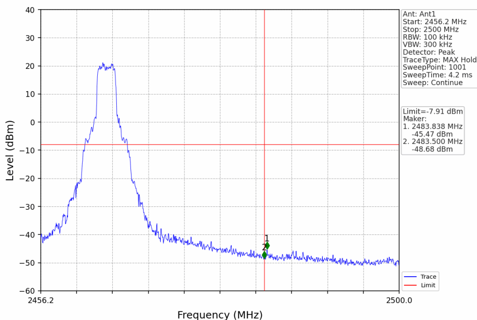
3M_HCH_2464.2MHz_Ant1_NTNV
