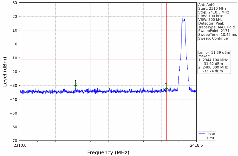
3M_LCH_2410.5MHz_Ant0_NTNV
