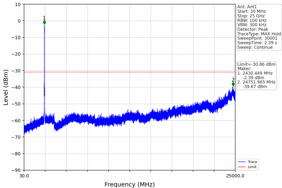
40M_MCH_2437.5MHz_Ant1_NTNV
