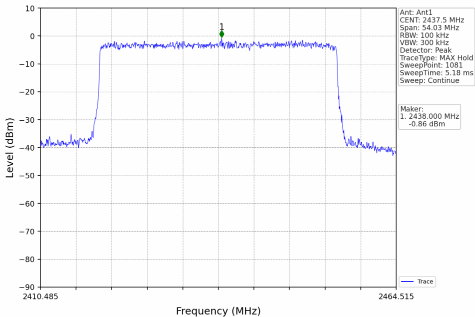
40M_MCH_2437.5MHz_Ant1_NTNV
