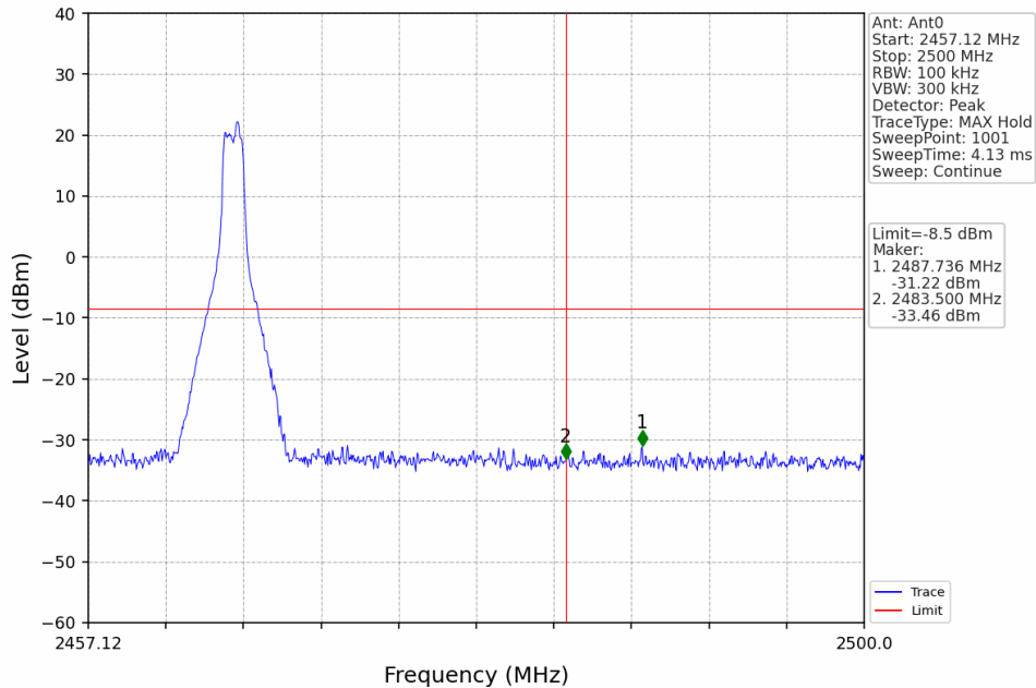
1.4M_HCH_2465.12MHz_Ant0_NTNV
