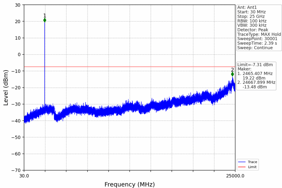
1.4M_HCH_2465.12MHz_Ant1_NTNV
