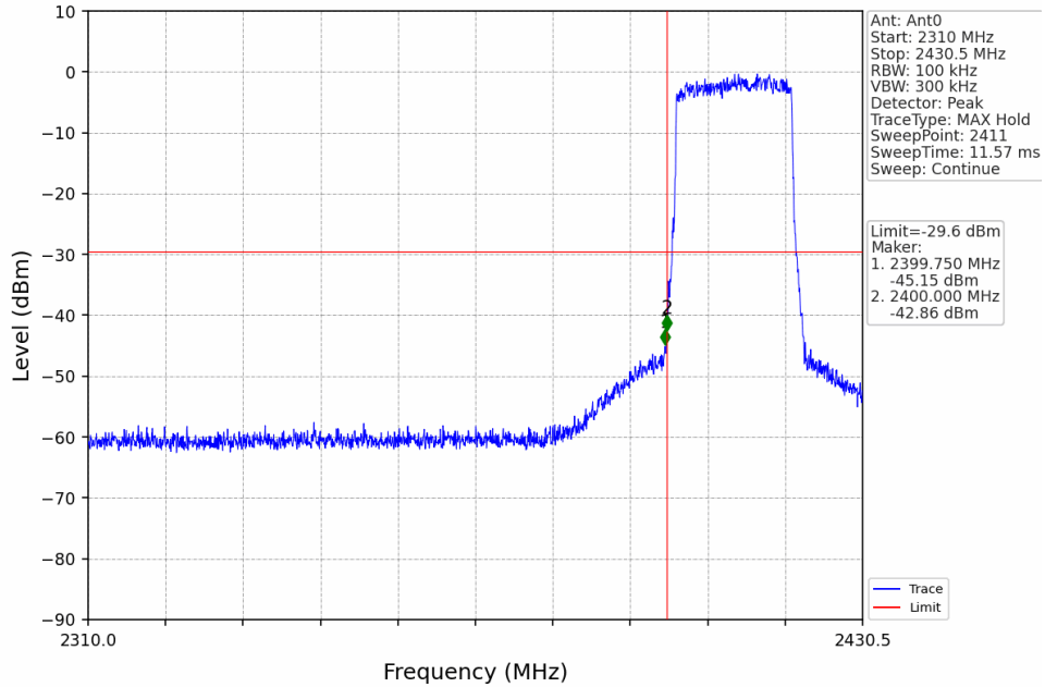
20M_LCH_2410.5MHz_Ant0_NTNV
