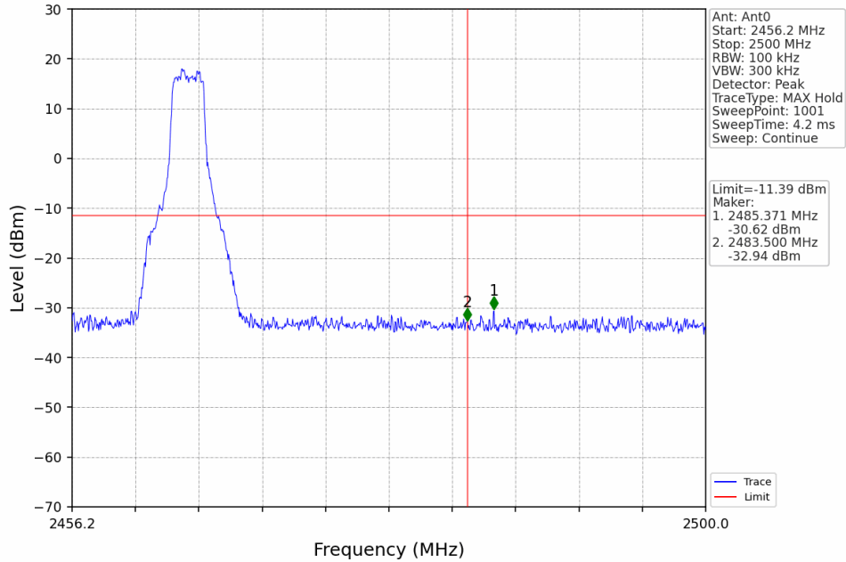
3M_HCH_2464.2MHz_Ant0_NTNV
