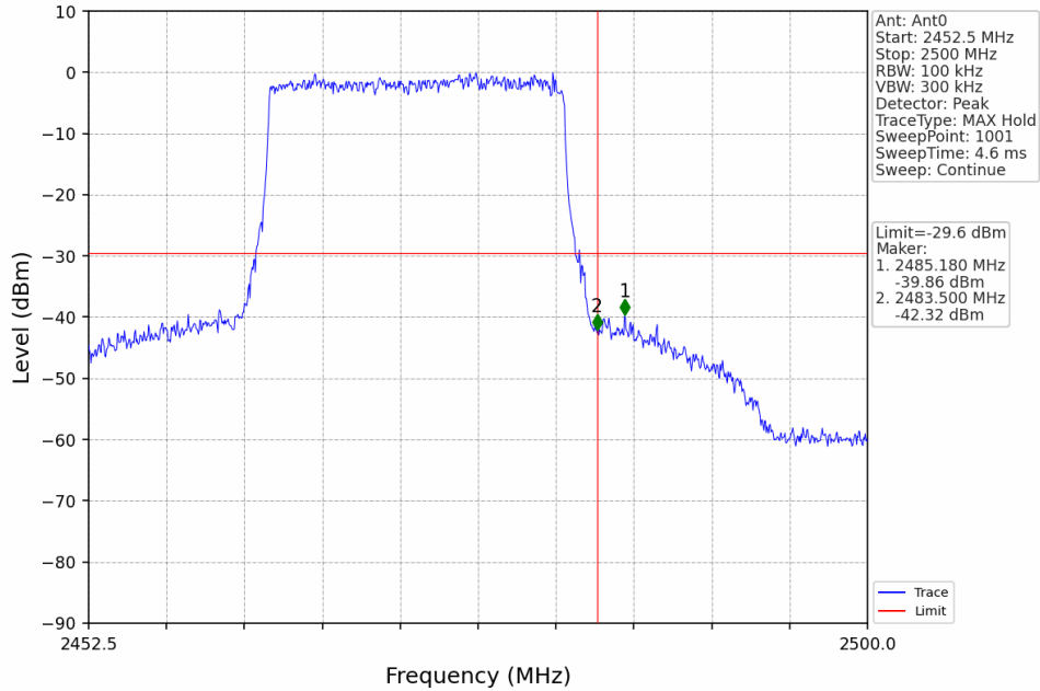
20M_HCH_2472.5MHz_Ant0_NTNV
