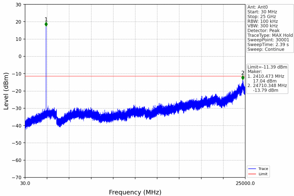
3M_LCH_2410.5MHz_Ant0_NTNV
