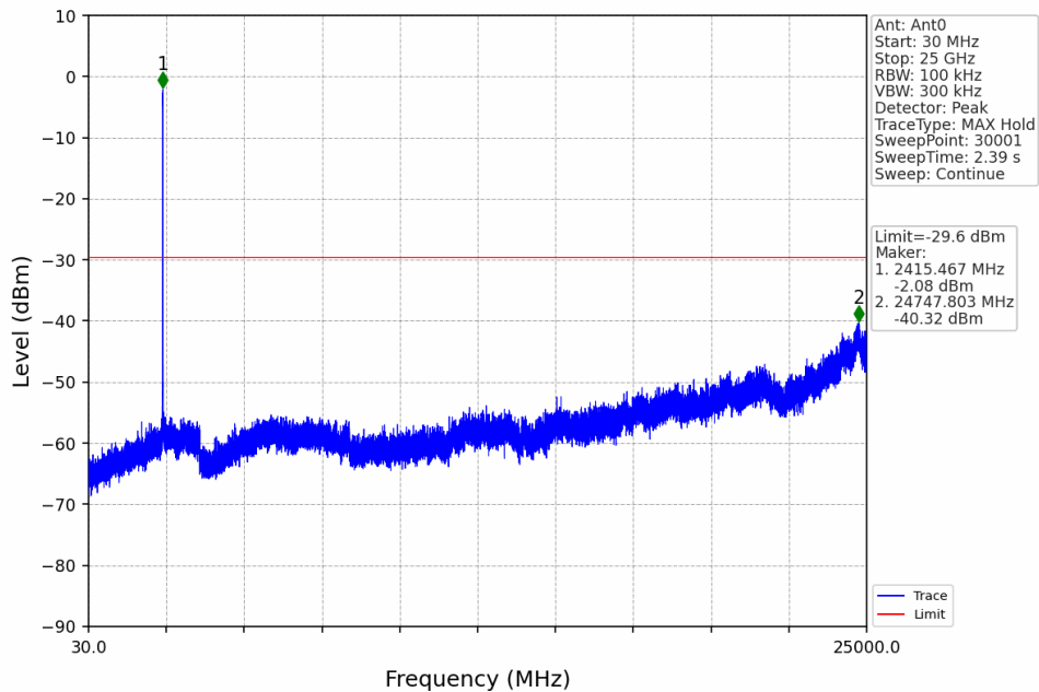
20M_LCH_2410.5MHz_Ant0_NTNV
