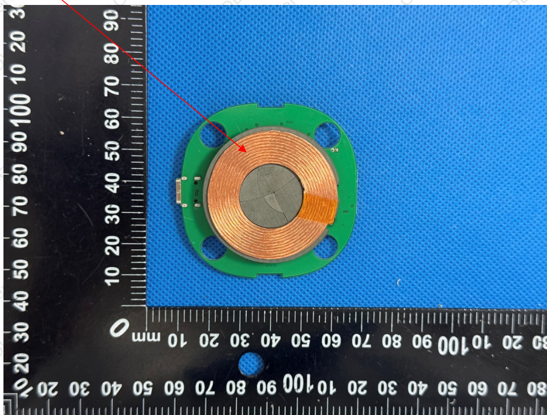
Antenna
