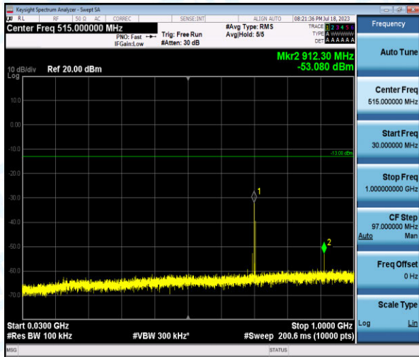
Band12-3MHz-QPSK-23095-1-0-Low-30-1000--53.08-PASS
