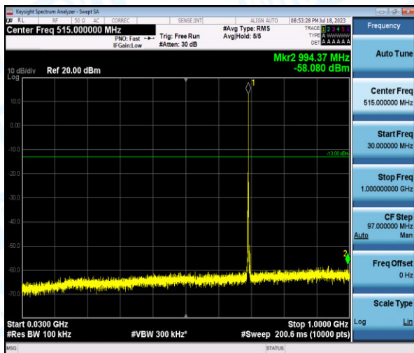
Band12-5MHz-QPSK-23035-1-0-Low-30-1000--58.08-PASS
