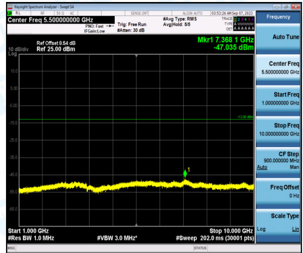
Band13-5MHz-16QAM-23230-1-0-Low-1000-10000--47.04-PASS
