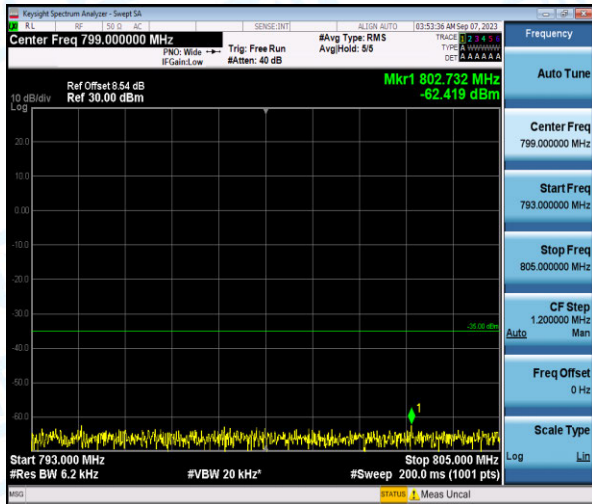
Band13-5MHz-16QAM-23230-1-0-Low-793-805--62.42-PASS
