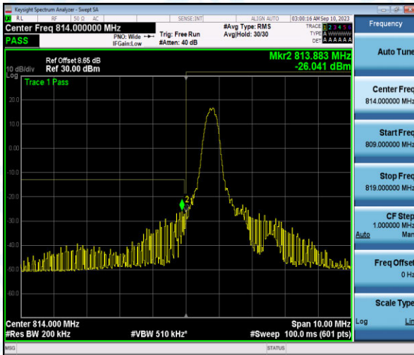
Band26-10MHz-QPSK-26740-1-0-Low--26.84,-26.04-PASS
