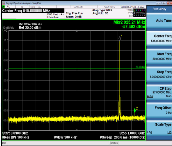
Band26-1.4MHz-QPSK-26740-1-0-Low-30-1000--57.49-PASS
