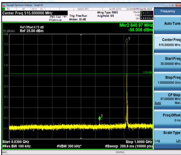
Band26-10MHz-QPSK-26840-1-0-Low-30-1000--58.01-PASS
