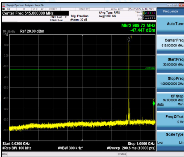
Band5-5MHz-QPSK-20425-1-0-Low-30-1000--47.45-PASS
