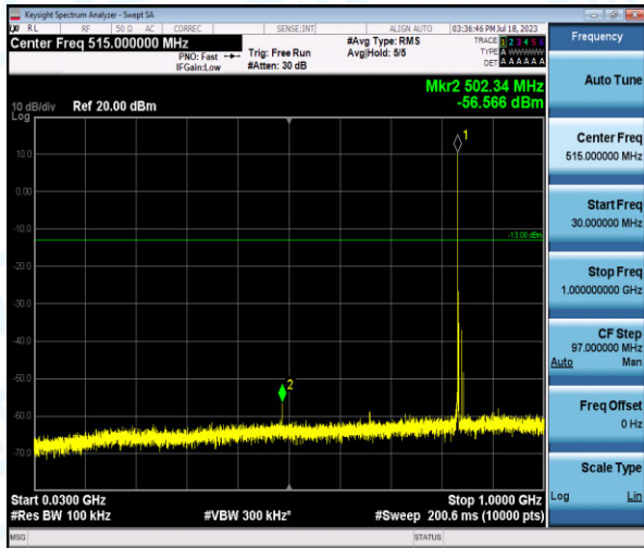
Band5-1.4MHz-QPSK-20525-1-0-Low-30-1000--56.57-PASS
