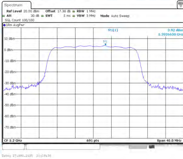
11AX20MIMO-Ant1-5200-PASS
