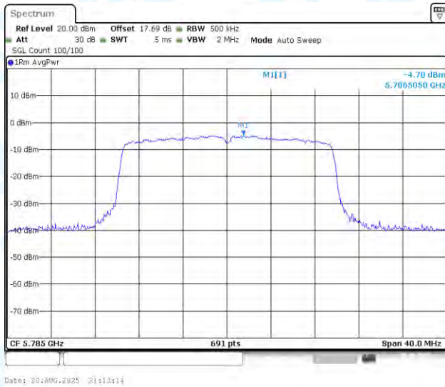
11AX20MIMO-Ant1-5785-PASS
