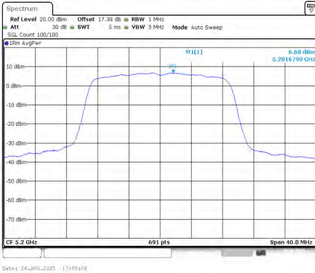
11N20MIMO-Ant1-5200-PASS
