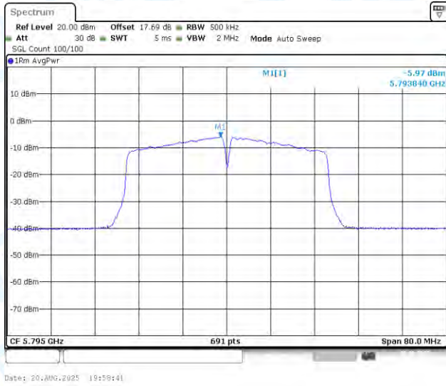
11N40MIMO-Ant1-5795-PASS
