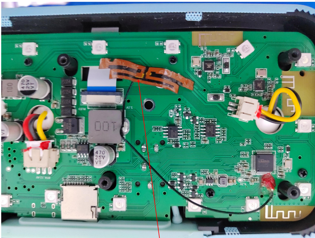
ANT 1
