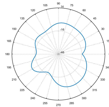
Phi_Polar_E2_5.5GHz
