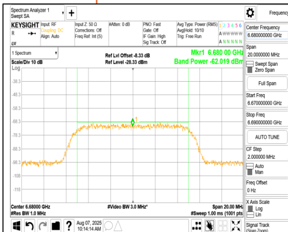
FMCW 150MHz 6750MHz AWGN:6680MHz
