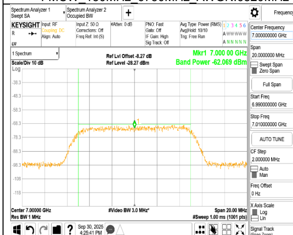
FMCW 150MHz 7000MHz AWGN:7000MHz
