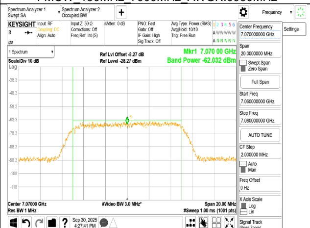
FMCW 150MHz 7000MHz AWGN:7070MHz
