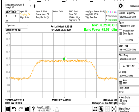
FMCW 150MHz 6750MHz AWGN:6820MHz
