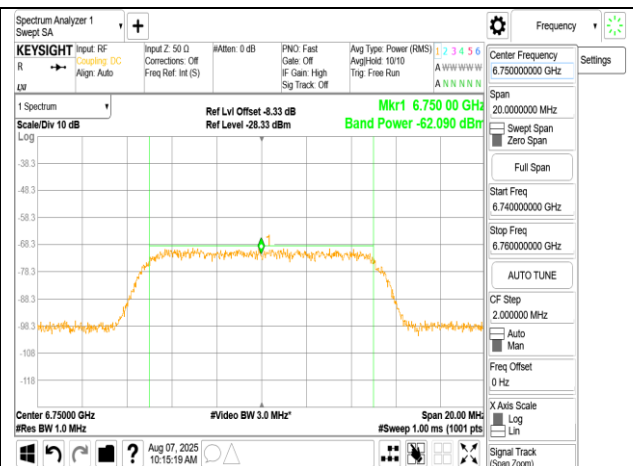
FMCW 150MHz 6750MHz AWGN:6750MHz
