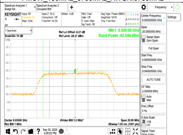
FMCW 150MHz 7000MHz AWGN:6930MHz
