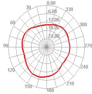
5150.000MHz E2
