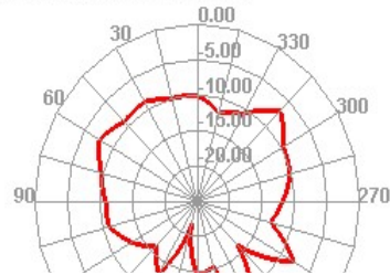
5150.000MHz E2
