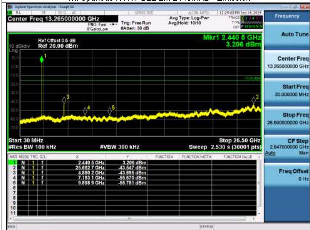
Tx. Spurious NVNT BLE 2M 2440MHz Emission
