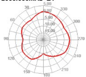
2500.000MHz E1
