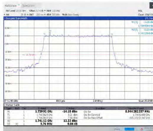
1-N66-PC3-15-10-M-4-DFT-64QAM-Outer_Full- 50@0-Ant1-8.944-9.760≤10-PASS
